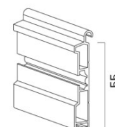
in allum. 14 x 55 ad inversione 55 mm
