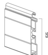
in allum. 14 x 55 55 mm
